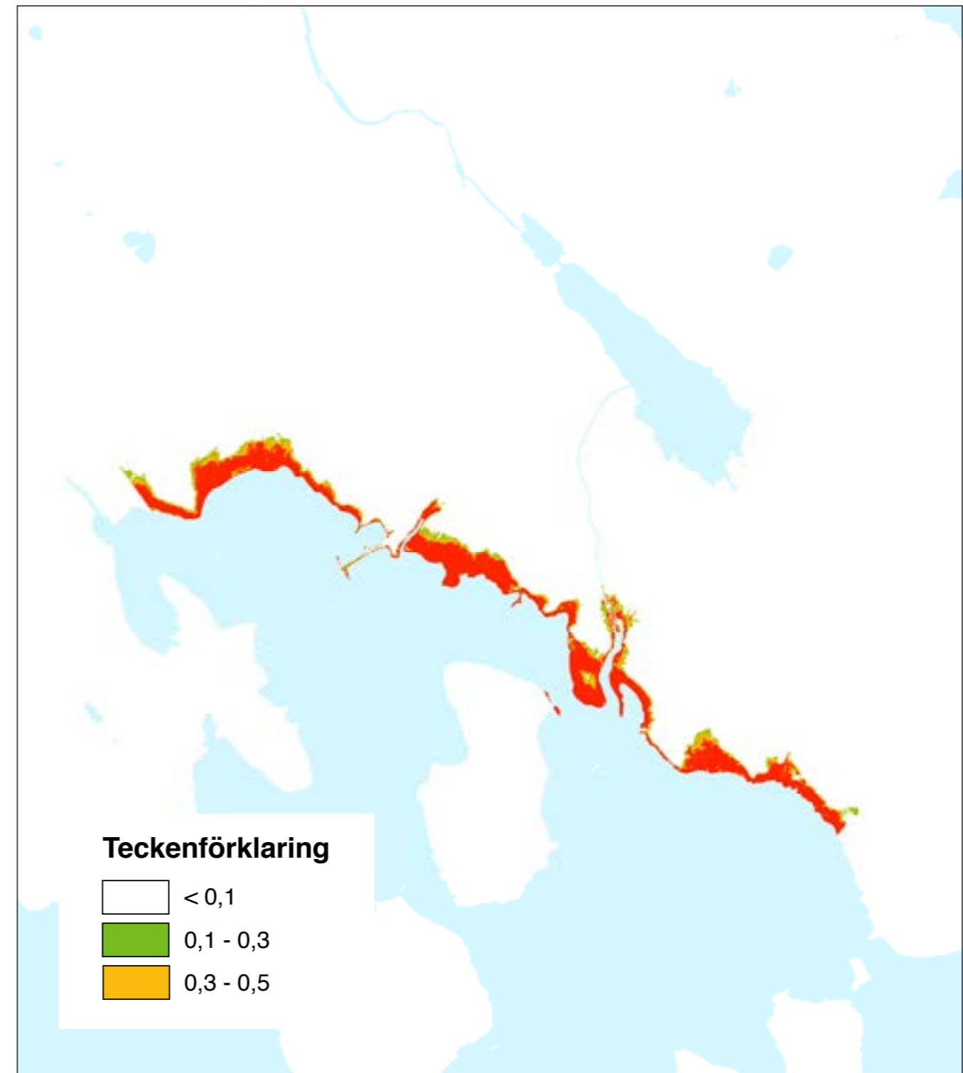
Simulerade översvämningsmodeller vid kraftiga skyfall; 100-årsstorm.
