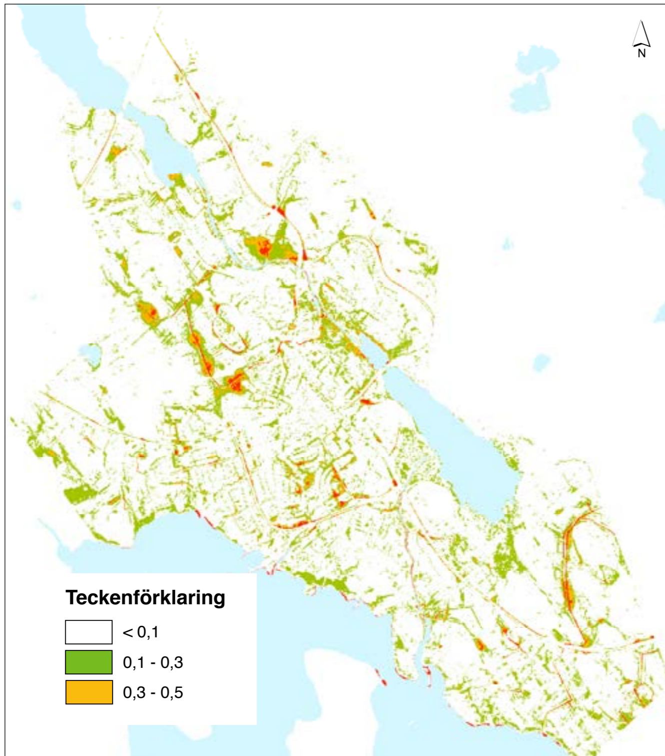
Simulerade översvämningsmodeller vid kraftiga skyfall; framtida 100-årsregn
