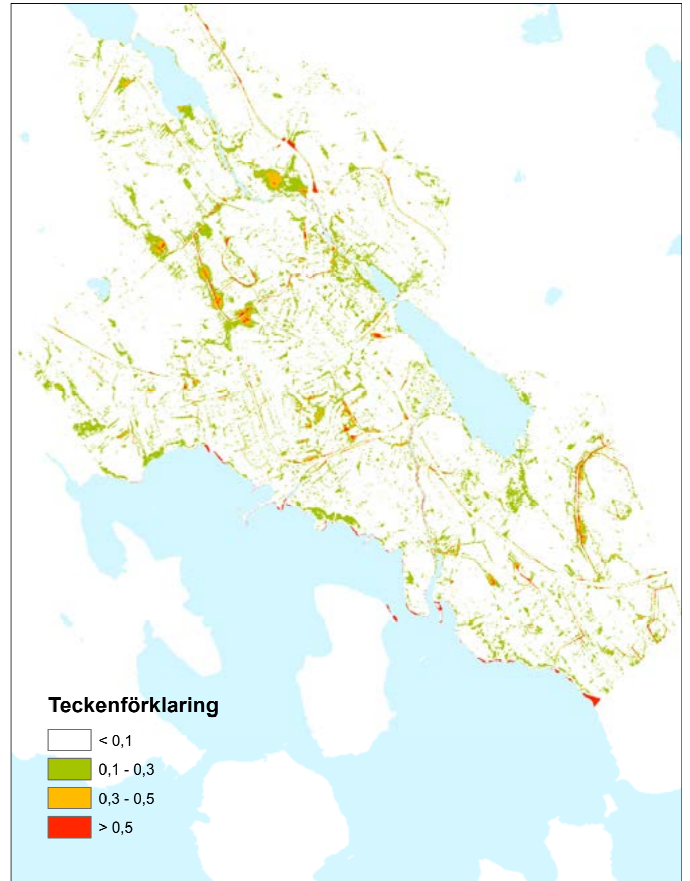
Simulerade översvämningssmodeller vid kraftiga skyfall; dagens 100-årsregn, framtida 100-årsregn samt 100-årsstorm.
