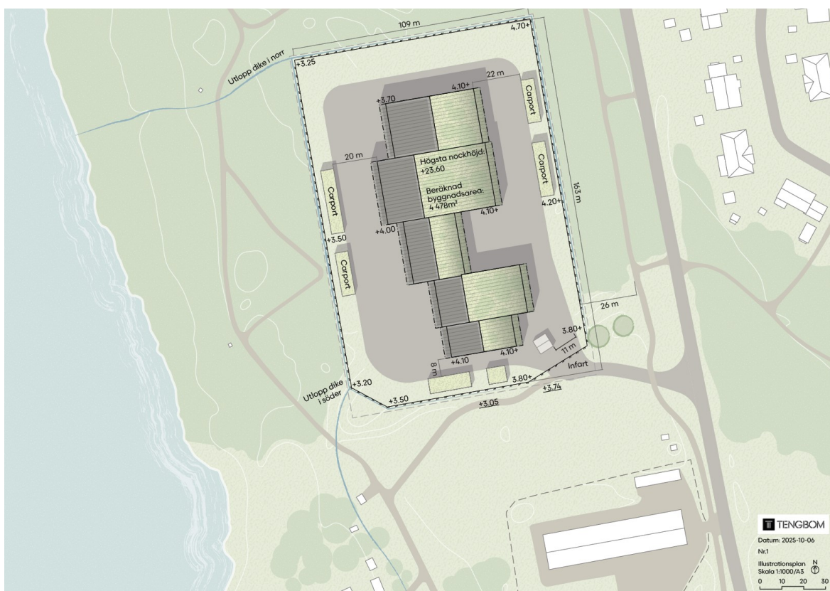
Figur 2. Illustration: Exempel som visar hur det nya vattenverket och området runt omkring kan komma att se ut. Källa: Gestaltungsdocument Piteå vattenverk (Tengbom, 2025-10-07).
