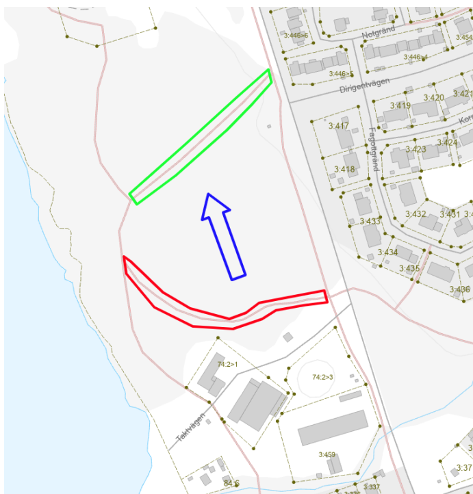
Figur 21. Förslag på ledningsflytt av elledning och belysning för gång- och cykelväg. Rödmarkerad GC-väg försvinner i och med detaljplanens genomförande och nytt läge för belysning samt ledning föreslås vid grönmarkerad GC-väg.
