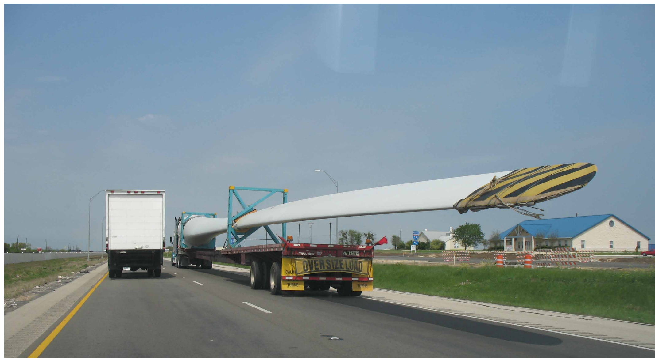
Transport av rotorblad på väg.
