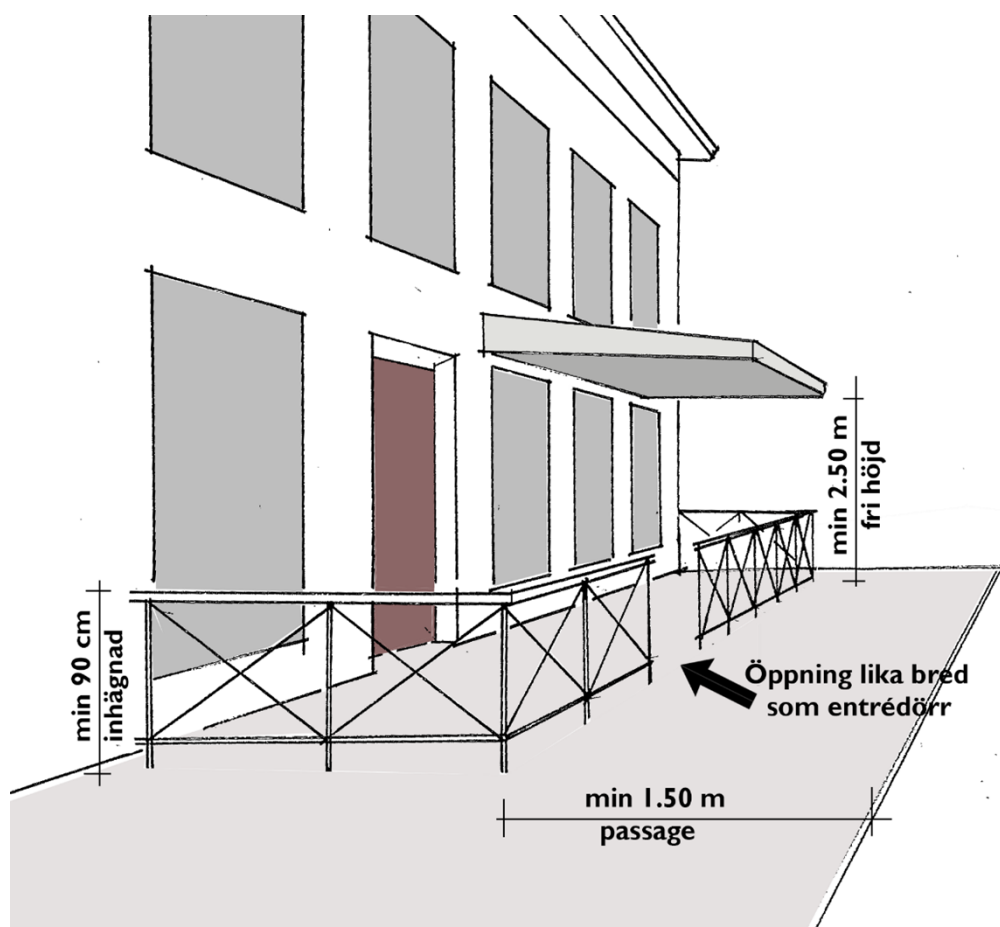
Bild 1: Illustrationen visar måttangivelser för placering, inhägnad och markiser
