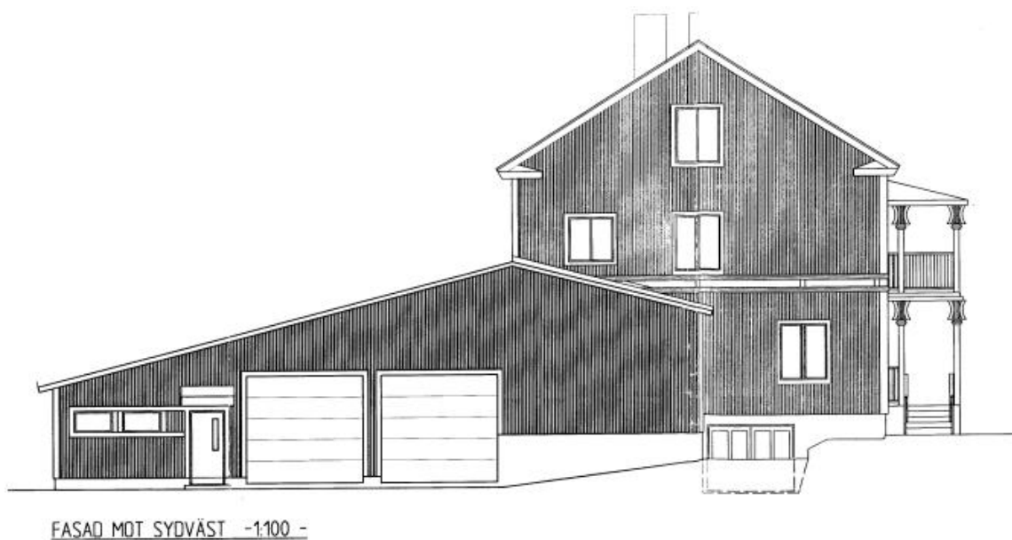
Figur 14. Bygglövsritning Pastorsexpeditionen.
