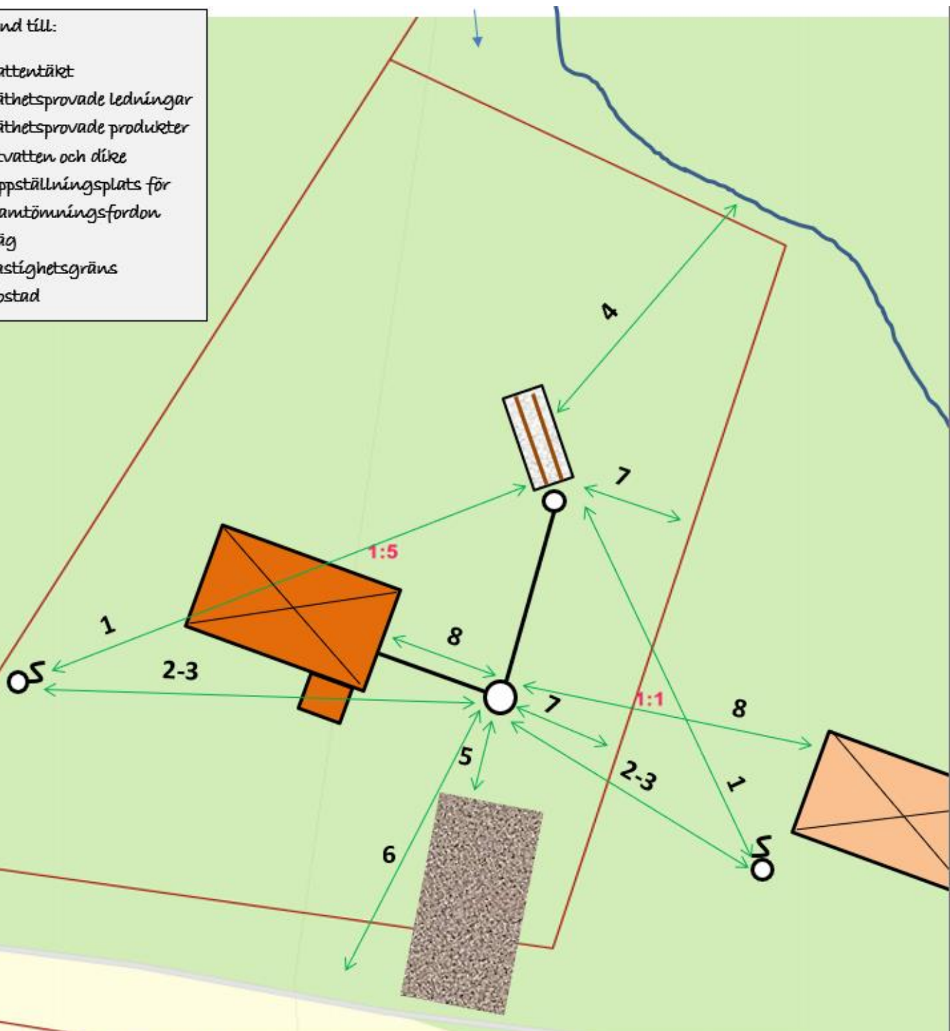
Figur 2. Horisontella skyddsavstånd
