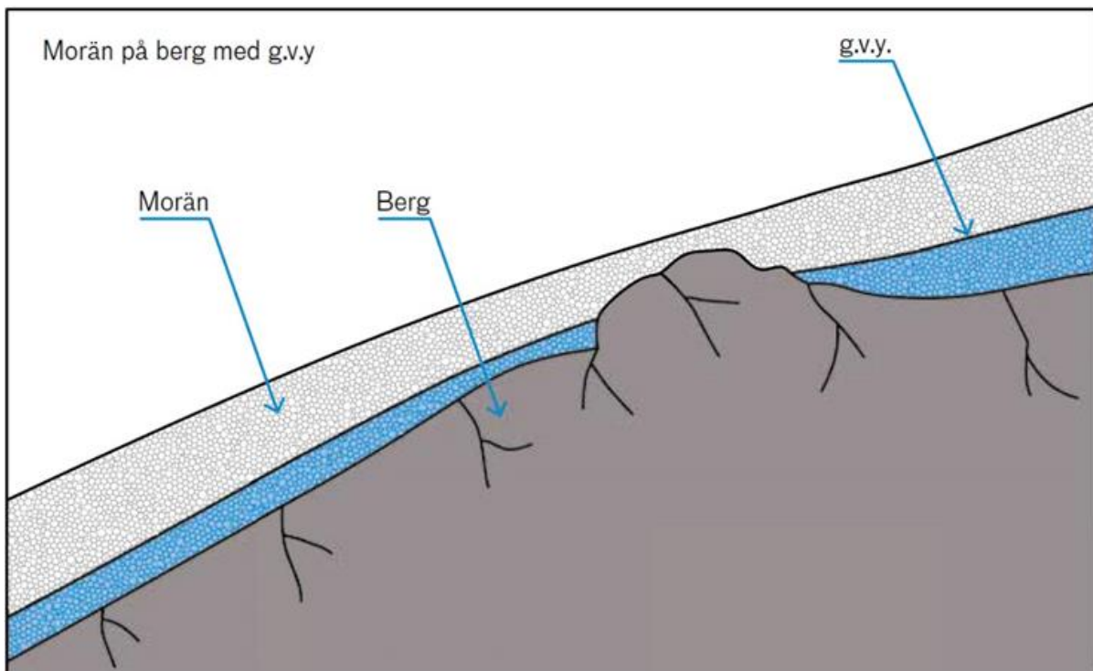
Figur 3. Om det är begränsat djup till berg finns anledning att undersöka utbredningen av olika jordlager. Då behöver man gräva flera provgroppar. G.v.y. är förkortning för grundvattenyta.
