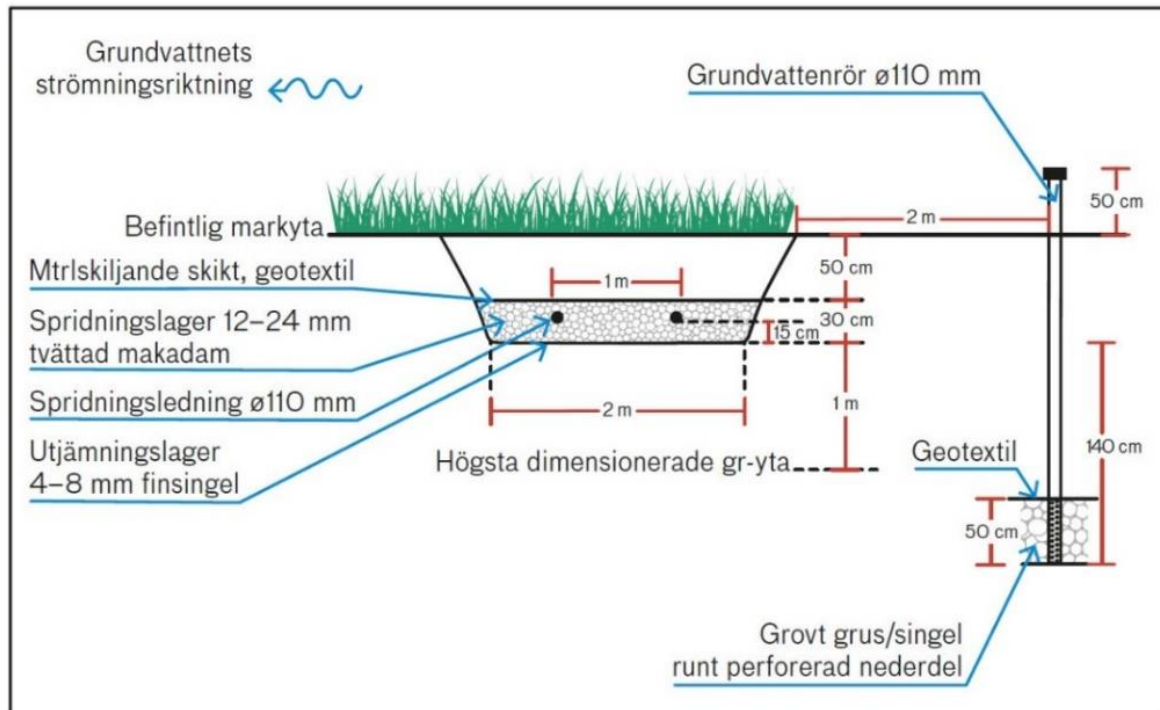
Figur 2. Exempel på tvärsektionsritning över infiltration med grundvattenrör för kontroll av grundvattennivå. Rörbotten bör ligga minst 140 cm under infiltrationsnivån (undre kanten på spridningslagret i detta exempel). Bifoga en tvärsektionsritning som underlag för installationsarbetet till din ansökan.
