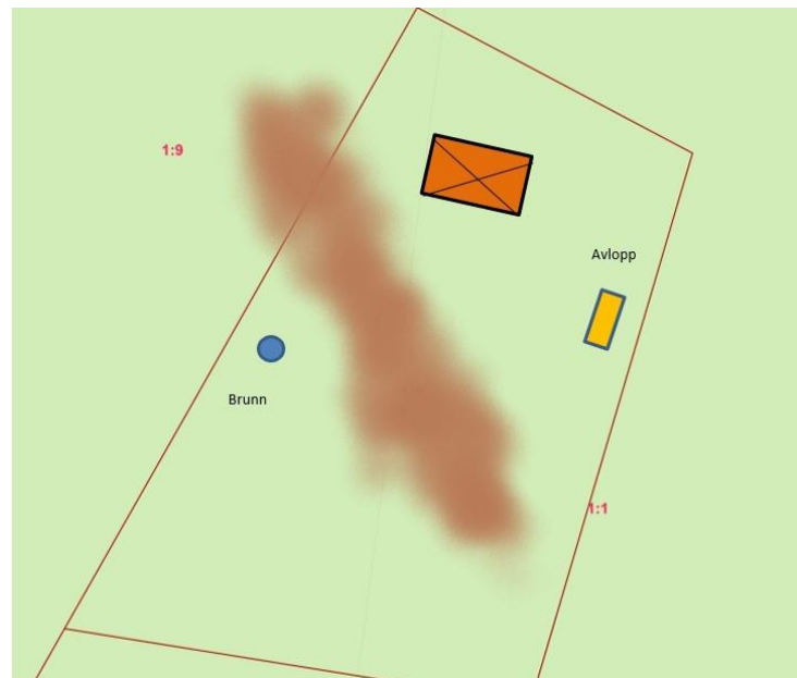
Figur 1 Berghällar mellan avlopp och dricksvattenbrunn, vilket begränsar avloppsvattnets möjlighet att sprida sig mot brunnen.
