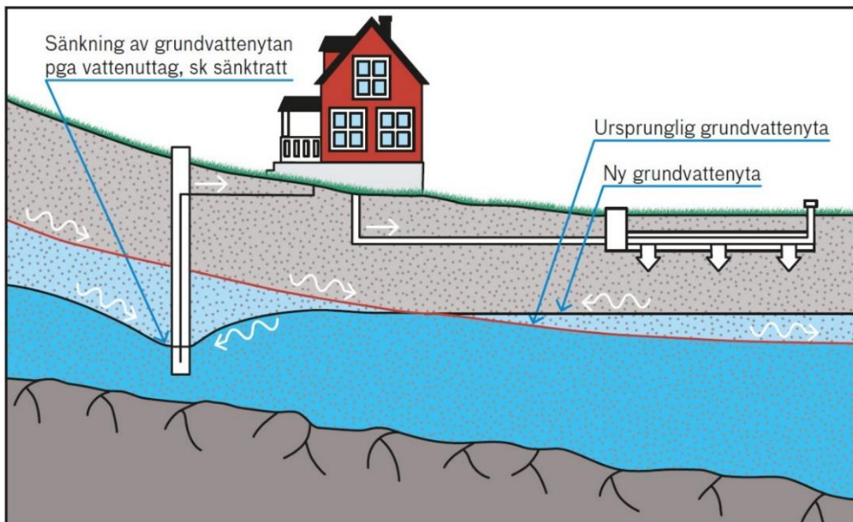
Figur 4. Vattentäkt och avloppsanläggning kan ändra grundvattnets strömningsriktning.
