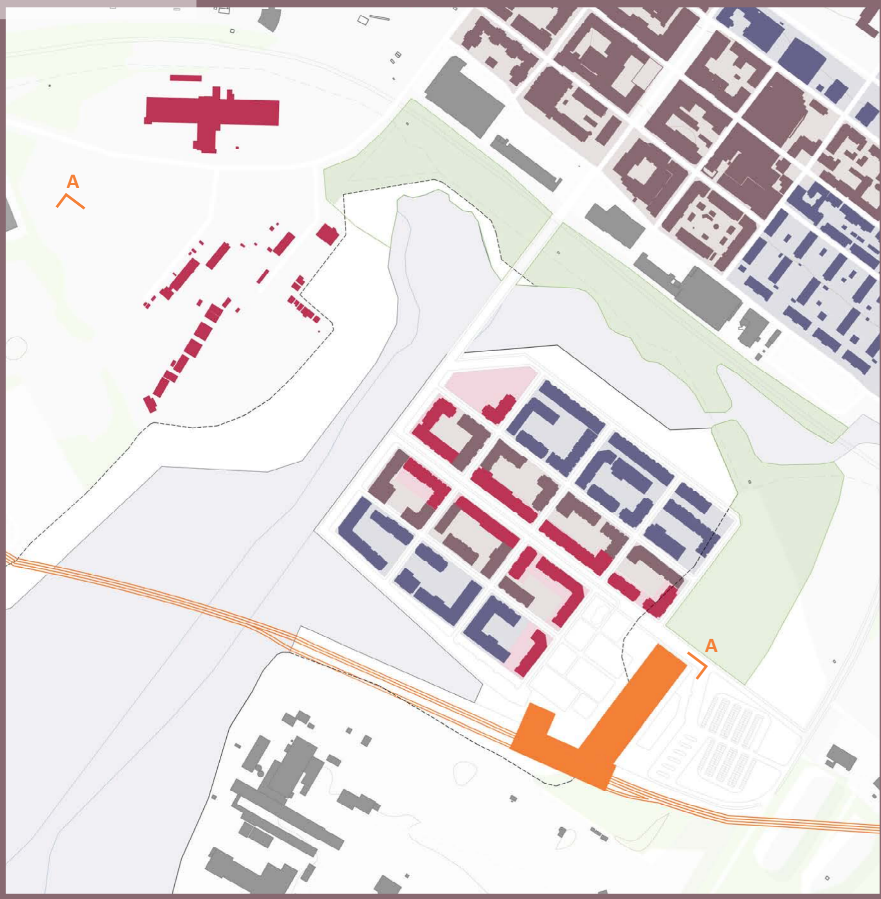
SITEPLAN 1:5000 0 50 100 (1)
